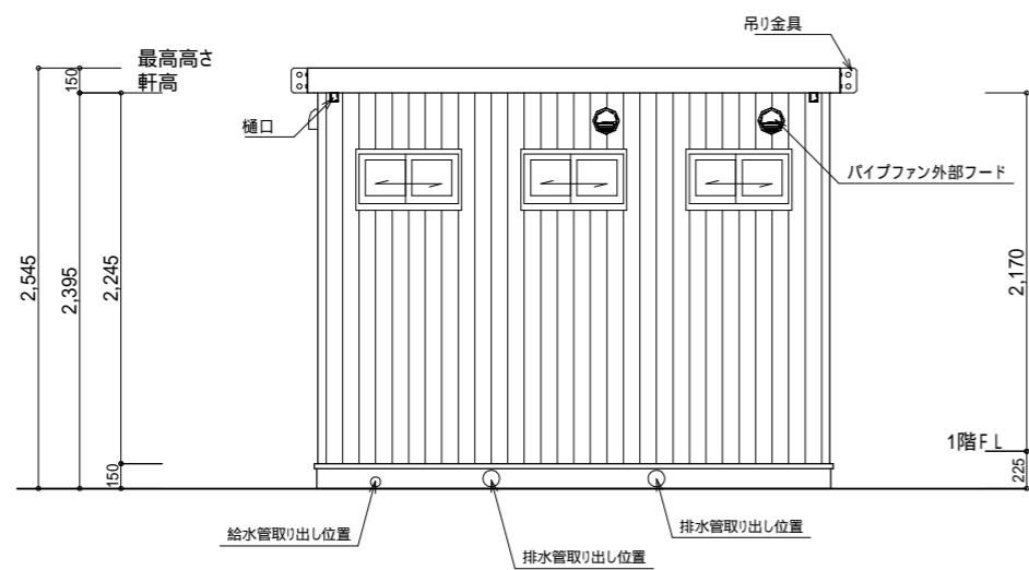
C側立面図 S:1/50
